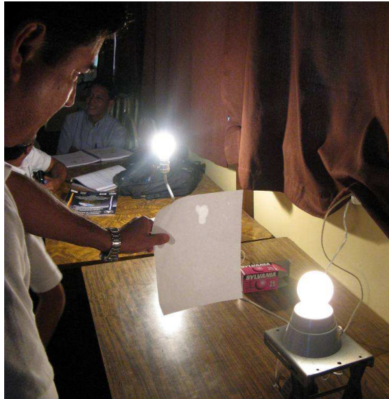
Fig. 16: Fotómetro de mancha de aceite, entre dos bombillas.
