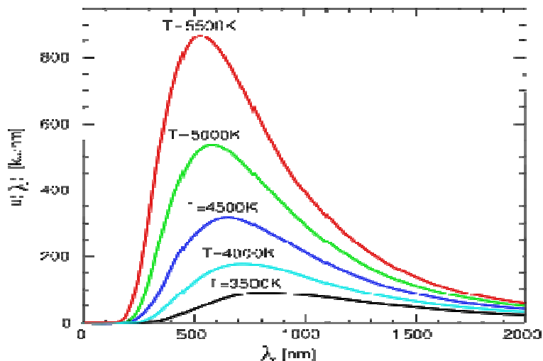
Fig. 21: Curvas de Planck de cuerpos negros a diferentes temperaturas.
