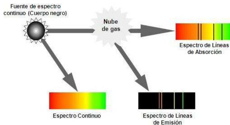
Fig. 19: Leyes de Kirchhoff y Bunsen
