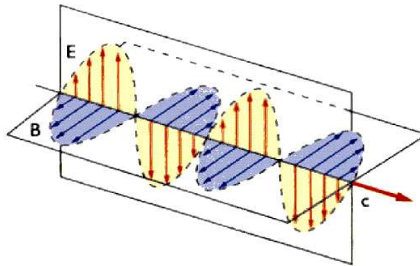
Fig. 2: Luz polarizada
